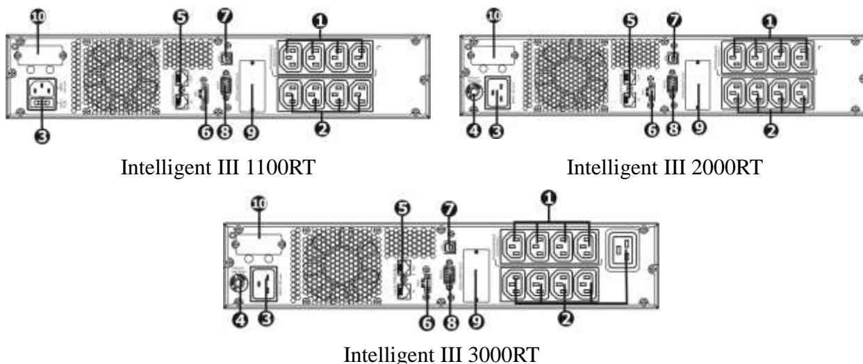
Рис. 2.2 Внешний вид задней панели ИБП
